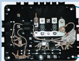
Sicherungsgehäuse | Fuse housing
