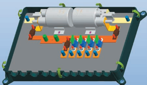
Sicherungsgehäuse / Energieverteiler Fuse housing / Power-Distribution-Board
