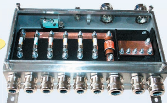
Hochvolt-Sicherungsbox High-Voltage-Fusebox
