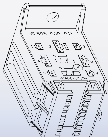
Belegung Relaishalter Allocation relay holder
