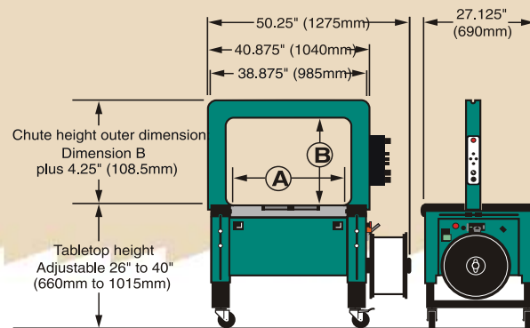
HBX-4330 Chute inner dimensions
